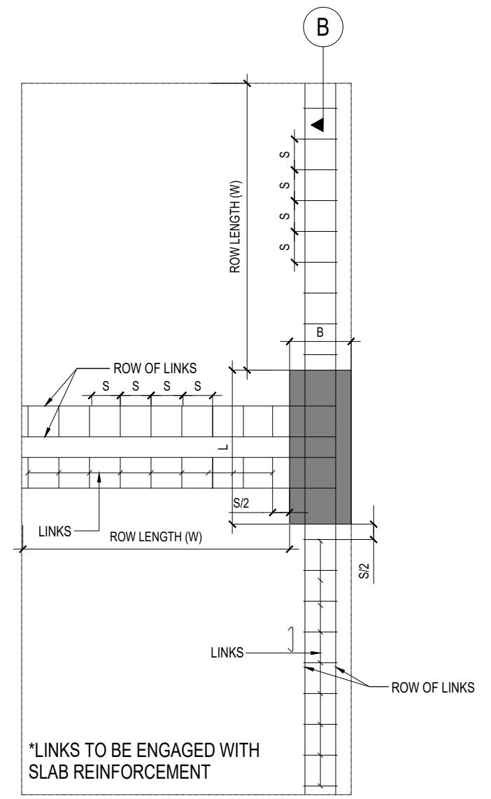
EDGE COLUMNS
